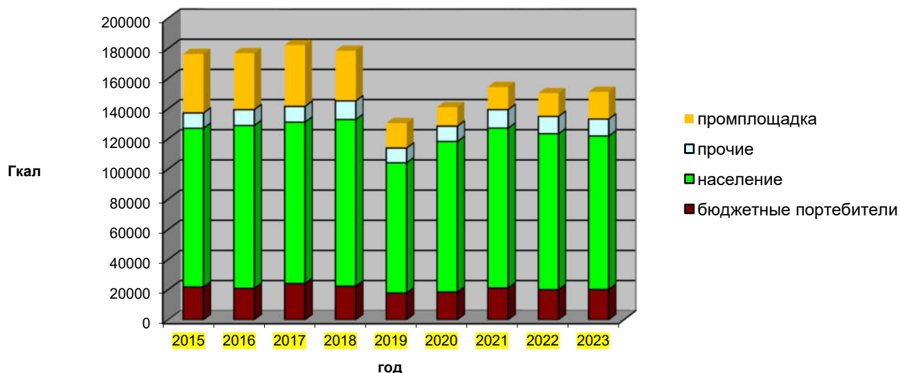
Диаграмма 2.1.5.4. Объем и структура потребления тепловой энергии
