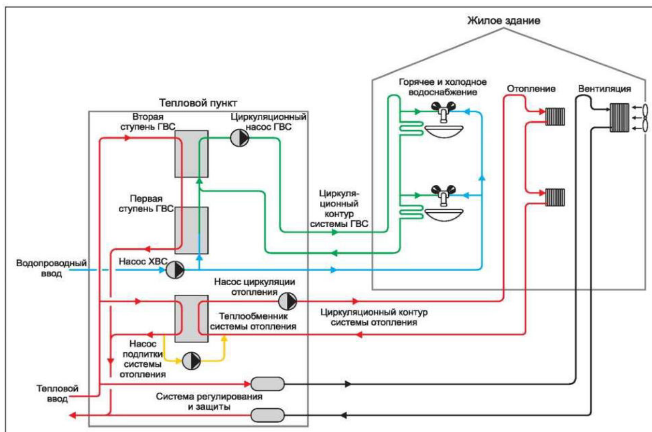
Рисунок 2.9.1. Принципиальная схема ТП с закрытой системой горячего водоснабжения и независимой схемой присоединения системы отопления
