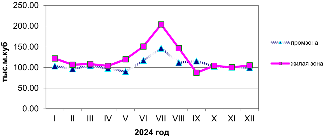
Диаграмма 3.2.3. Объемы подачи артезианской воды централизованными системами водоснабжения МО г.Яровое в 2024 г.
